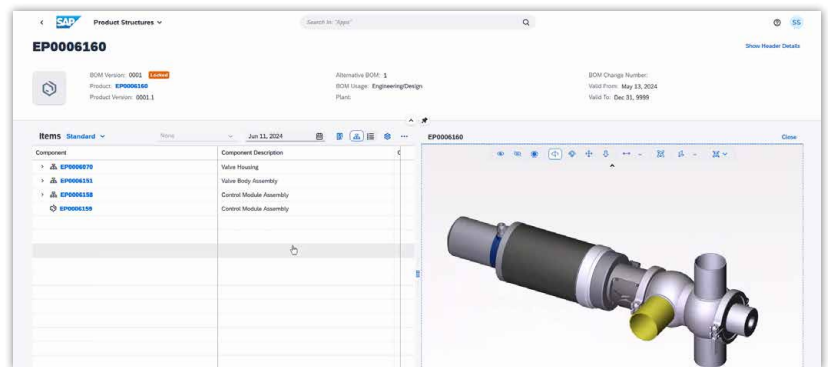
Solid Edge Baugruppe als SAP Product Structure dargestellt – inklusive Visualisierung
