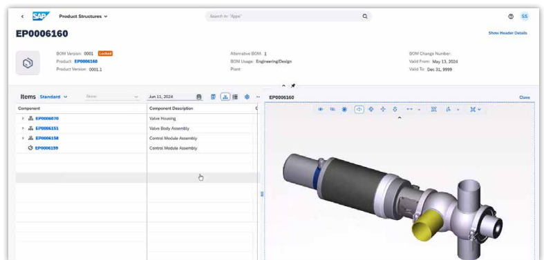
SOLIDWORKS Baugruppe als SAP Product Structure dargestellt – inklusive Visualisierung
